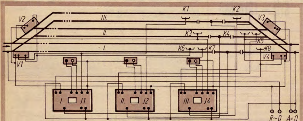
I. KAPCSOLÁS
